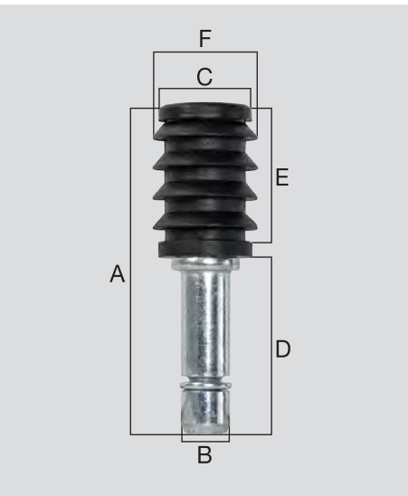
Stift verzinkt, mit Rundrohrhülse Ø 17 mm Galvanised stem, with round cap Ø 17 mm Tige zinguée, avec douille ronde Ø 17 mm
