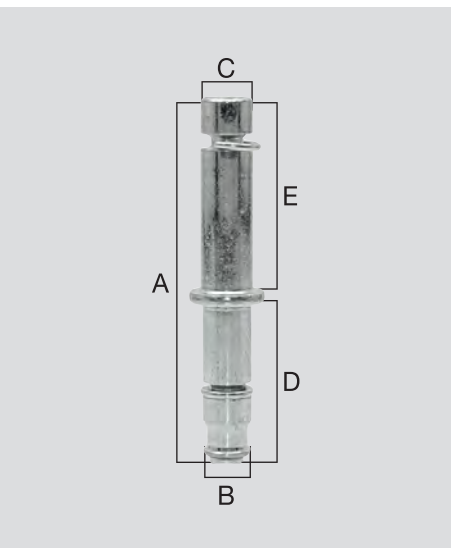
Reduzierstift verzinkt Ø 8,5 mm Galvanised reducing stem Ø 8,5 mm Tige à réduire zinguée Ø 8,5 mm
