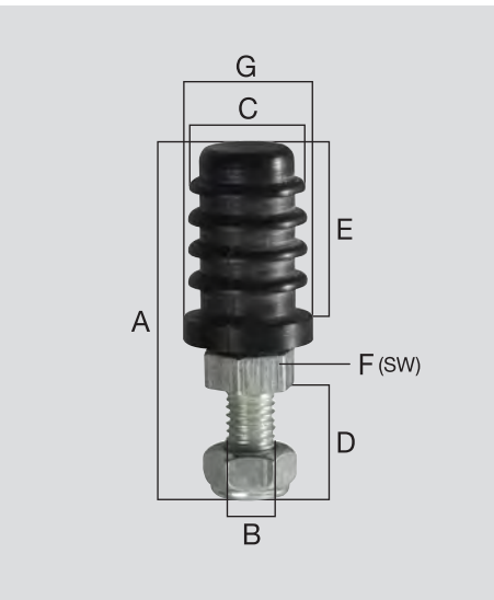
Stift verzinkt, mit Rundrohrhülse Ø 17 mm / Ø 20 mm Galvanised stem, with round cap Ø 17 mm / Ø 20 mm Tige zinguée, avec douille ronde Ø 17 mm / Ø 20 mm
