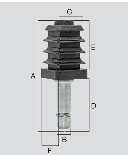
Stift verzinkt, mit Vierkanthülse 17 x 17 mm Galvanised stem, with square cap 17 x 17 mm Tige zinguée, avec douille carrée 17 x 17 mm
