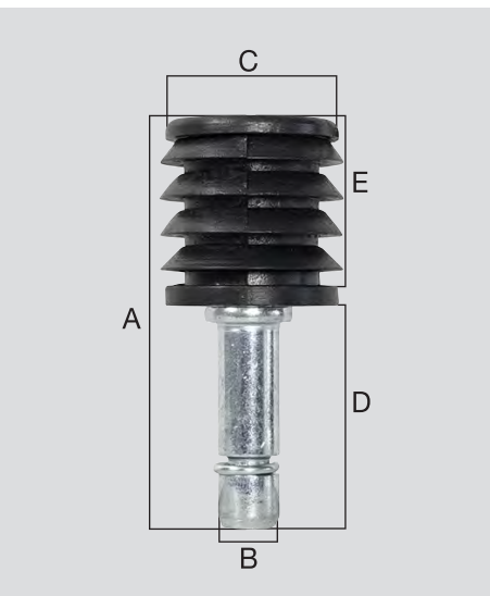
Stift verzinkt, mit Rundrohrhülse Ø 22 mm Galvanised stem, with round cap Ø 22 mm Tige zinguée, avec douille ronde Ø 22 mm
