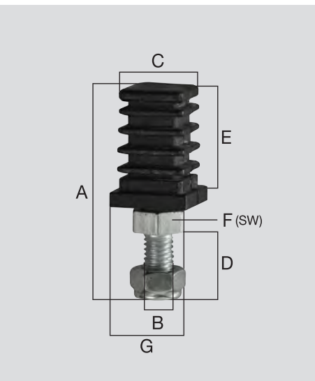
Stift verzinkt, mit Vierkanthülse 17x17mm / 20x20mm Galvanised stem, with square cap 17x17mm / 20x20mm Tige zinguée, avec douille carée 17x17mm / 20x20mm
