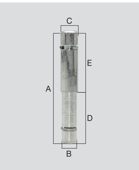
Reduzierstift verzinkt Ø 9 mm Galvanised reducing stem Ø 9 mm Tige à réduire zinguée Ø 9 mm
