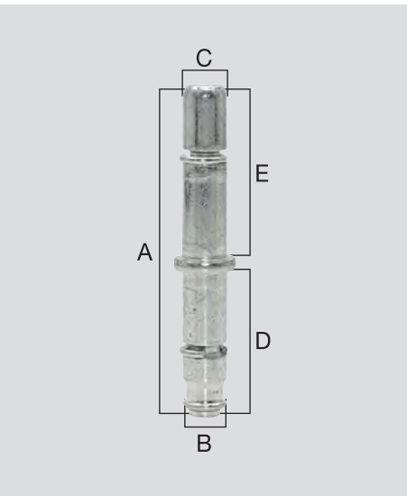
Steckstift verzinkt Ø 8 mm Galvanised insert stem Ø 8mm Tige zinguée Ø 8 mm
