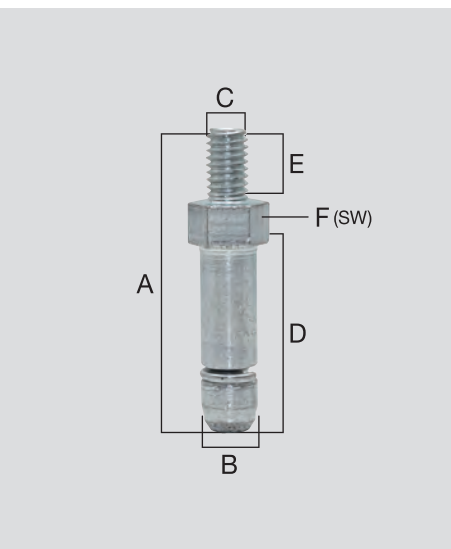
Gewindestift verzinkt M 6 x 8 mm / SW 10 mm Galvanised threaded stem M 6 x 8 mm / SW 10 mm Tige filetée zinguée M 6 x 8 mm / SW 10 mm
