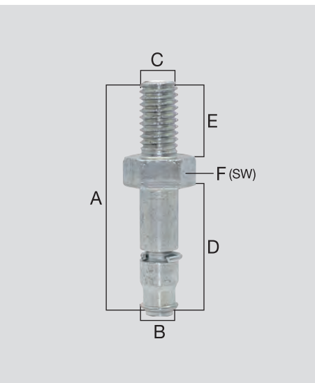
Gewindestift verzinkt M 8 x 15 mm / SW 13 mm Galvanised threaded stem M 8 x 15 mm / SW 13 mm Tige filetée zinguée M 8 x 15 mm / SW 13 mm
