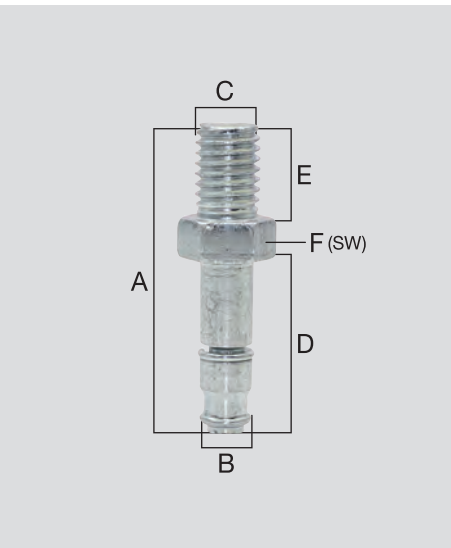
Gewindestift verzinkt M 10 x 14 mm / SW 13 mm Galvanised threaded stem M 10 x 14 mm / SW 13 mm Tige filetée zinguée M 10 x 14 mm / SW 13 mm
